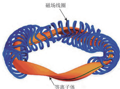
图2 仿星器中线圈配置
